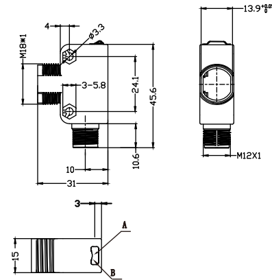
M12 连接器
