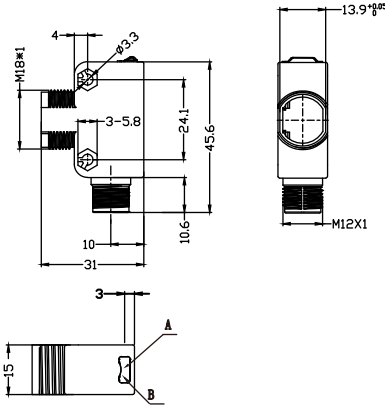
M12 连接器
